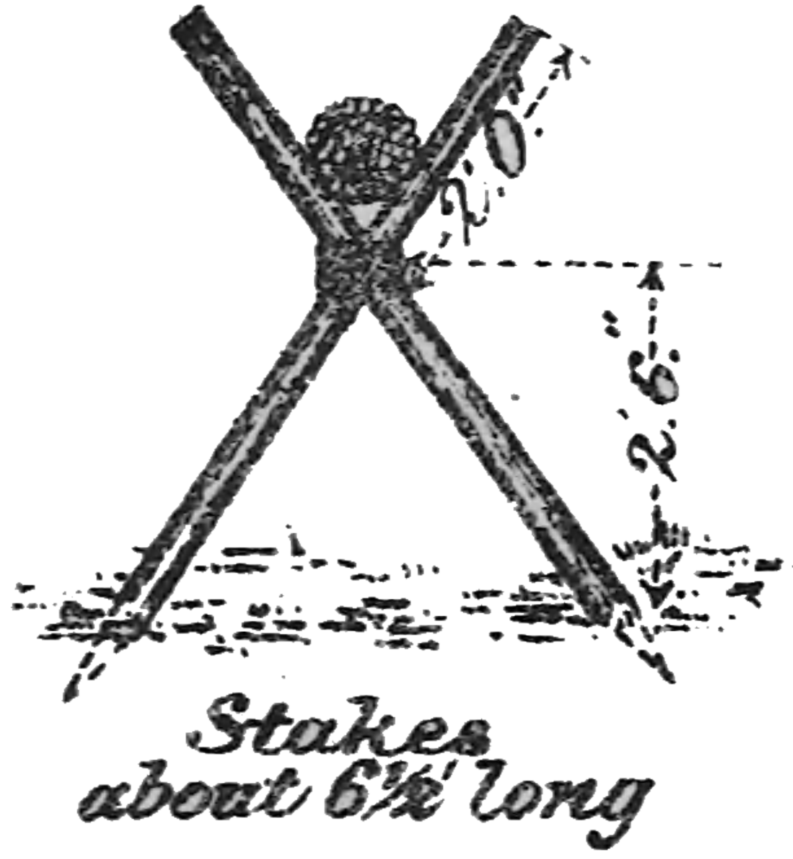
Fig. 6. Fascine Trestle
