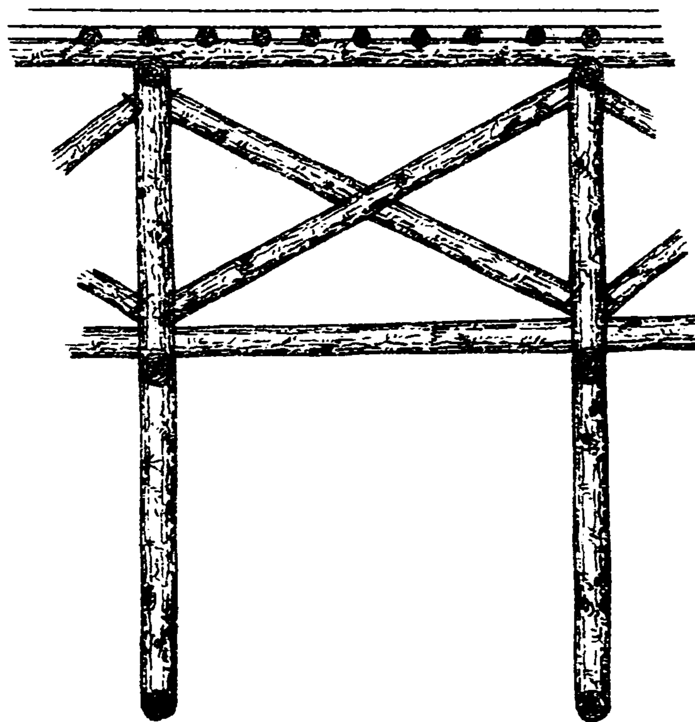
Elevation
